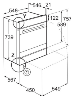
Einbaubackofen/Einbauherd EB7.../EH7...
